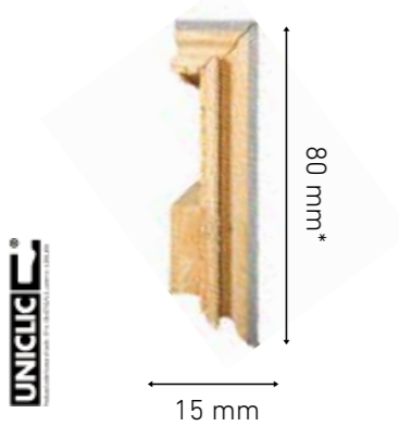
ZÓCALO CLIC CLASSIC (SUIZA)
