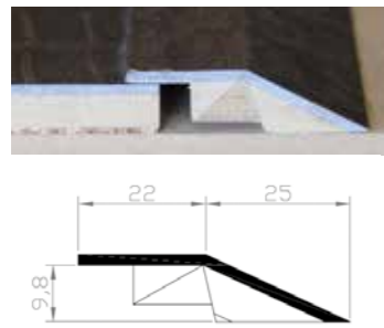
JUNTA DE TRANSICIÓN CON PAVIMENTO (SUIZA)
