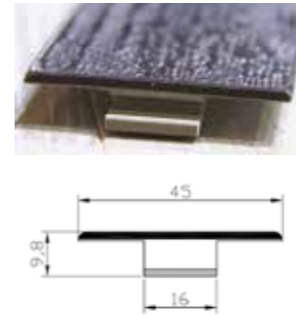
JUNTA DE DILATACIÓN CON PAVIMENTO (SUIZA)
